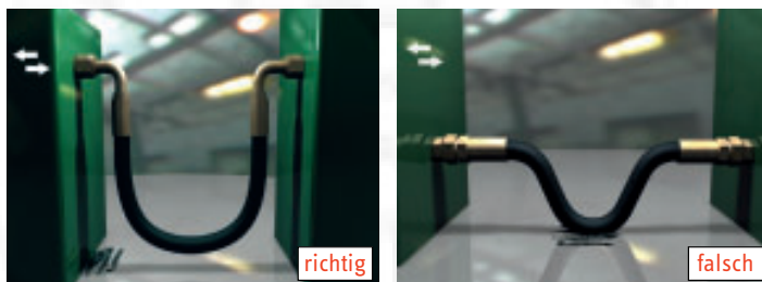
Abbildung 9: Vermeidung von Abrieb durch ausreichende Bewegungsfreiheit
